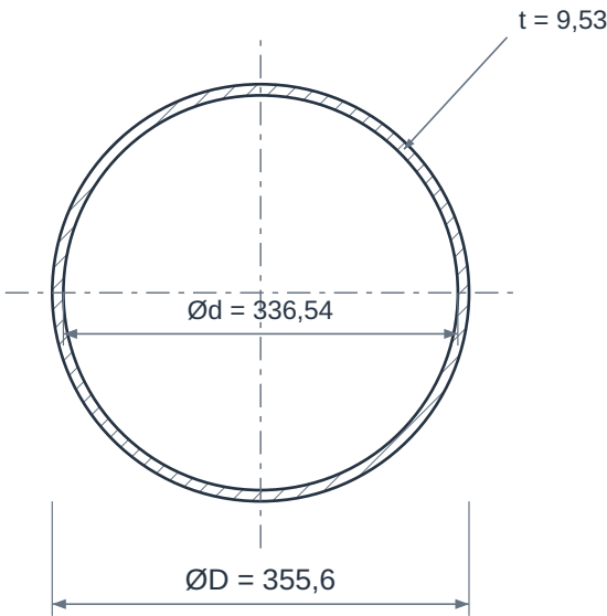
SEÇÃO A-A
