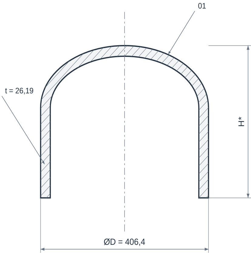
CORTE LONGITUDINAL
