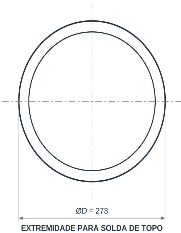
DETALHE DA EXTREMIDADE
